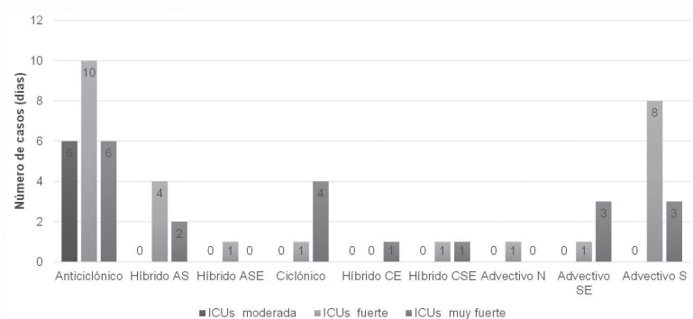
Figura N° 14 Número de días analizados con Terra MODIS según tipo de tiempo de J&C y categorías de ICUs.
